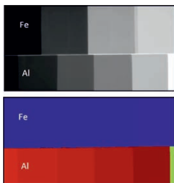
Fig. 8. Radiographic image (left) taken at 160kV and dual energy image (right) of Fe (blue) and Al (red) step wedges (green = free beam/air) [2] Rys. 8. Radiogram (z lewej) wykonany przy 160 kV i obraz dwuenergetyczny (z prawej) klinów schodkowych wykonanych z Fe (niebieski) i Al (czerwony) (barwa zielona = powietrze) [2]
