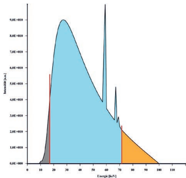
Fig. 7. Selective detection of a bremsstrahlung spectrum (example) by thresholding inside of the detector [2] Rys. 7. Selektywne wykrycie promieniowania hamowania (przykład) poprzez progowanie wewnątrz detektora [2]
