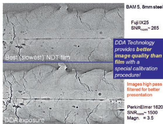
Fig. 9. Enhanced detail visibility of flaws by increased SNR of a DDA image in comparison to a digitized film image of weld sample BAM 5 after numeric high pass filtering [1] Rys. 9. Poprawiona widoczność detali wad na próbce spawu BAM 5 poprzez zwiększenie SNR obrazu otrzymanego z użyciem detektora cyfrowego, w porównaniu do obrazu otrzymanego ze zdigitalizowanego zdjęcia rentgenowskiego przetworzonego za pomocą cyfrowego filtru górnoprzepustowego [1]
