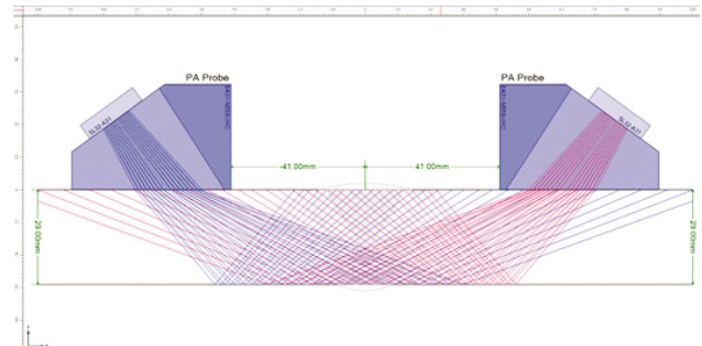
Rys. 1. Symulacja pokrycia wiązkami ultradźwiękowymi przy skanowaniu UTPA typu Compound dla kątów 40°–70° dla głowicy OLYMPUS 5L32 z klinem SA31 55°, aktywna apertura 16-elem (płyta o grubości 29 mm).
