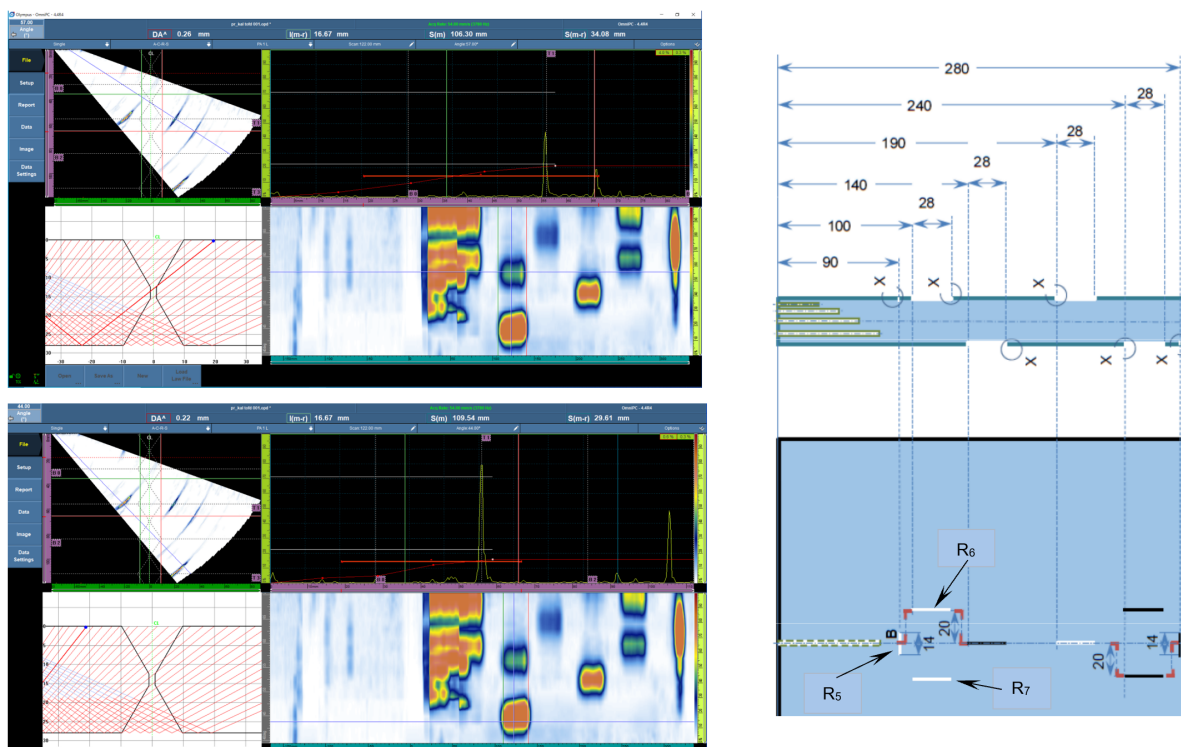
Rys. 10. Reflektory R_6 oraz R_7 – nacięcie w licu x_{6,7}=(100+28) mm; y_6=20 mm; (h \times w)_{6,7}=(1 \times 0,2) mm – skany PA(DS) dla próbki RB#28 od strony TOP. Skany TOFD „nie widzą” R_5 ; R_6 oraz R_7
