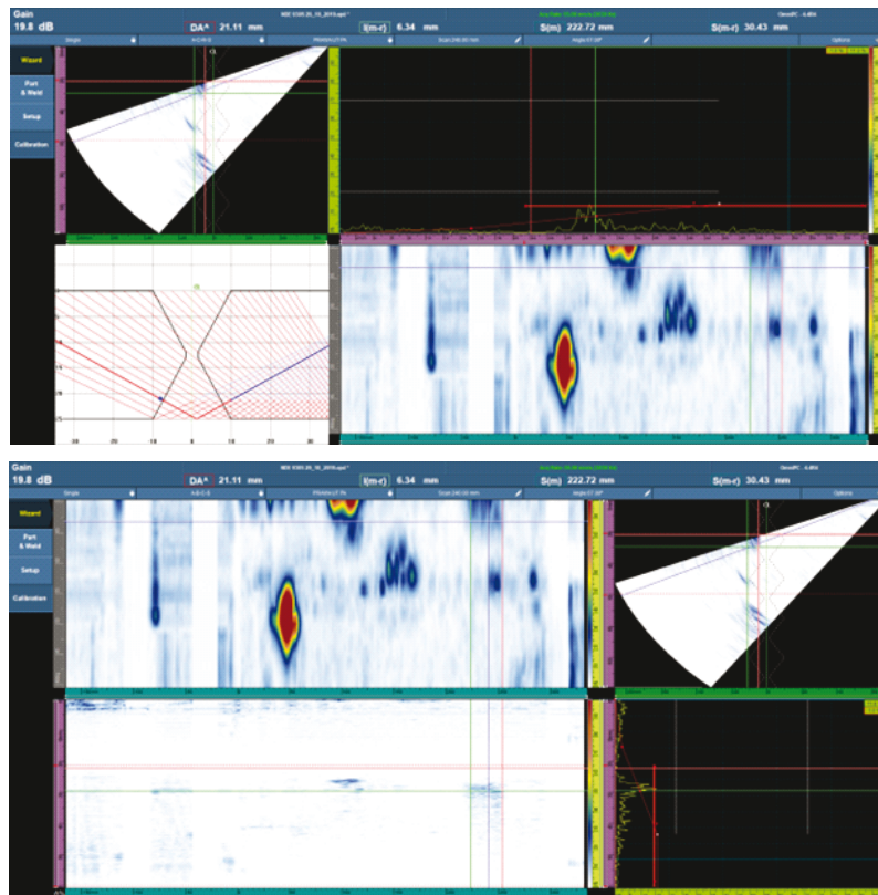
Rys. 19. Zobrazowania i wymiary tej wady ( x = 222,7 + 30,4 mm; z_3 = 21,1 mm) wg skanu próbki walidacyjnej głowicą PA(US).
