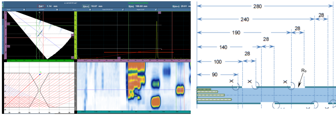
Rys. 12. Reflektor R_9 nacięcie w środku lica x_9 = (190 + 28) mm; y_9 = 0 mm; (h \times w)_9 = (1 \times 0,2) mm – wg skanu głowicą PA(DS) dla próbki RB#28 od strony TOP. Skany TOFD „nie widzą” R_9 .
