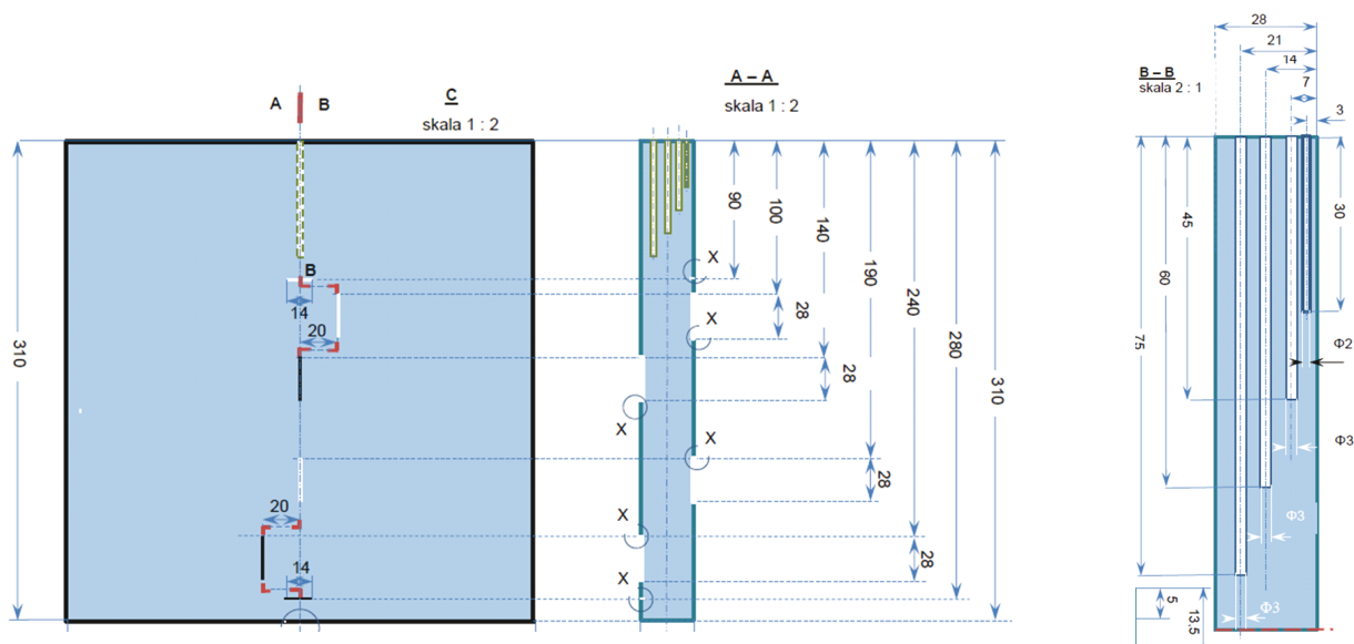
Rys. 4. Próbką odniesienia dla poziomu C, do weryfikacji nastaw systemu ultradźwiękowego PA+TOFD
