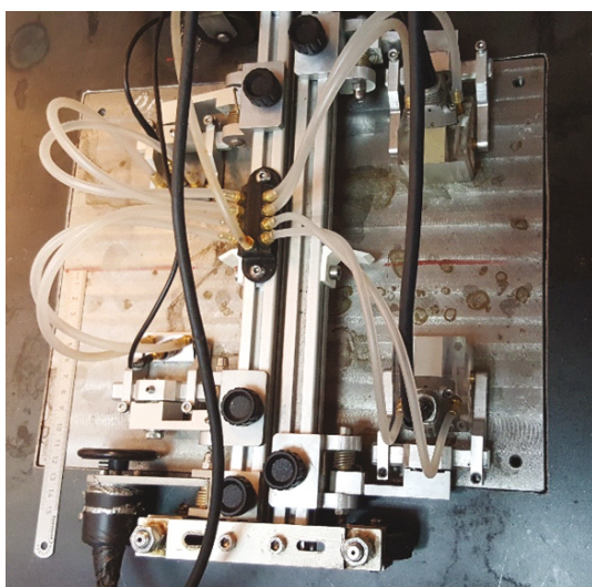
Rys. 2. Wygląd skanera PA+TOFD w wersji ręcznej.
