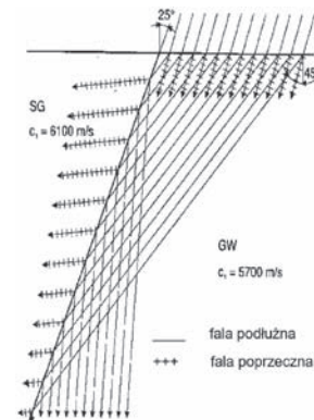
Rys. 8. Całkowite odbicie fali podłużnej od granicy wtopienia złącza austenitycznego
