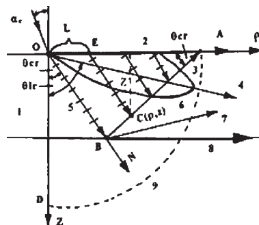
Rys. 15. Konfiguracja wiązek w głowicy fal podpowierzchniowych: 1. obiekt badany, 2. fala pełzająca I rodzaju, 3. front fali poprzecznej, 4. fala podłużna główna I rodzaju, 5. fala poprzeczna główna, 6. obwiednia listka głównego fali podłużnej, 7. fala podłużna główna II rodzaju, 8. fala pełzająca II rodzaju, 9. front fali podłużnej
