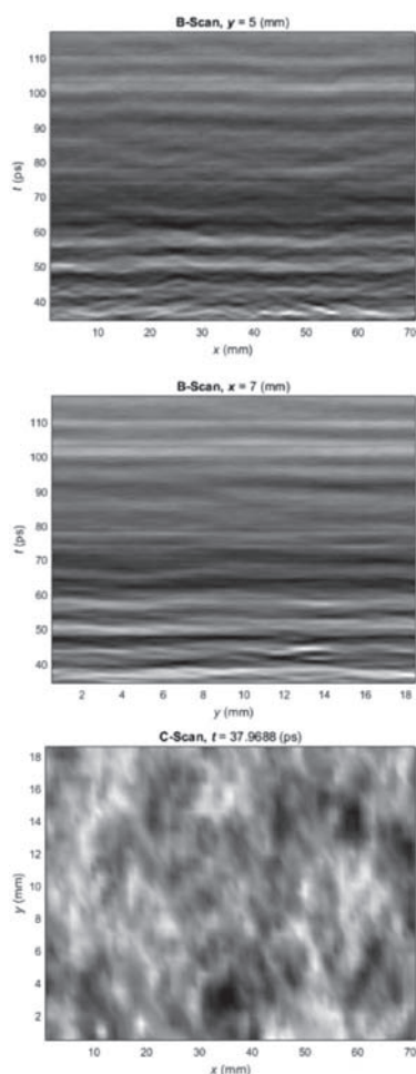
Rys. 10. Sygnały zmierzone dla próbki płyty włókno-cementowej „E”
