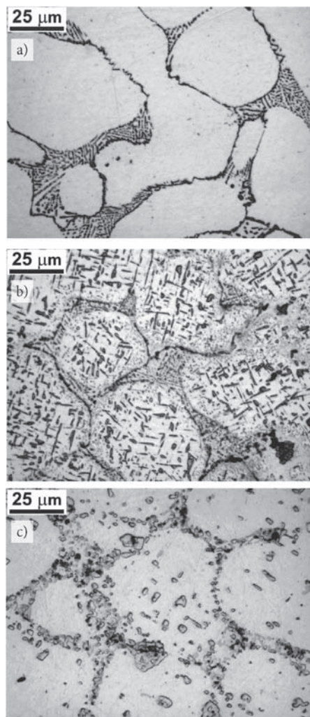
Rys. 5. Mikrostruktura IN519: a) stan lany, b, c) po 120 760 h eksploatacji [17]
