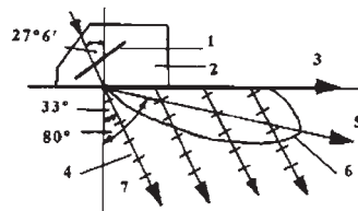
Rys. 14. Zasada tworzenia fal w głowicy fal podpowierzchniowych: 1. przetwornik 2. głowica 3. fala pełzająca I rodzaju – fala podłużna (primary creeping wave) 4. fala poprzeczna główna 5. fali podłużna główna 6. obwiednia listka głównego fali podłużnej 7. Fale poprzeczne wtórne
