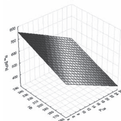
Rys. 6. Zależność wytrzymałości na rozciąganie staliwa IN 519 od parametru Larsona-Millera i twardości Brinella rur w reformerach Z.Ch. „POLICE”
