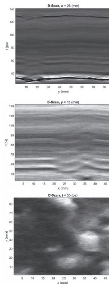
Rys. 11. Sygnały zmierzone dla próbki płyty włókno-cementowej z defektami sztucznymi
