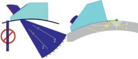
Fig. 4. Sectorial Scan view showing depth ruler not applicable Rys. 4. Obraz skanu sektorowego (S-skan) pokazuje nieaktualną liniijkę głębokości
