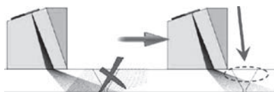
Rys. 13. W przypadku braku możliwości usunięcia lica wskazania wad w strefie przypowierzchniowej spoiny austenitycznej należy badać falą podłużną – L pełzającą, tzn. falą podpowierzchniową.
