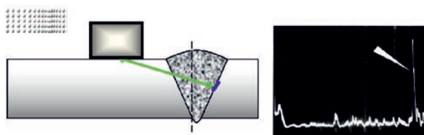
Rys. 12. Lokalizacja i obraz wskazania wady w spoinie austenitycznej falą podłużną – L
