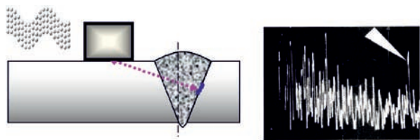
Rys. 11. Lokalizacja i obraz wskazania wady w spoinie austenitycznej falą poprzeczną spolaryzowaną pionowo – T_v
