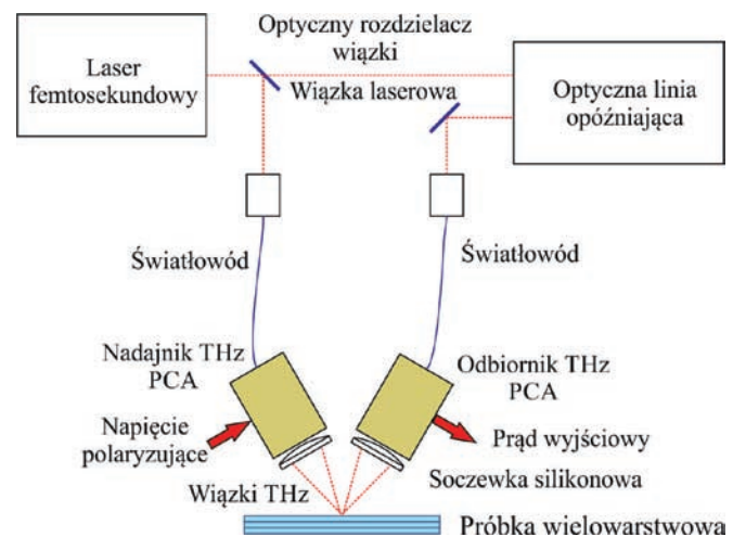
Rys. 3. Uproszczony schemat systemu teraherowego TDS pracującego w trybie odbiciowym w układzie z niezależnymi głowicami Fig. 3. Simplified scheme of the terahertz time domain spectroscopy working in reflection mode in configuration with independent heads
