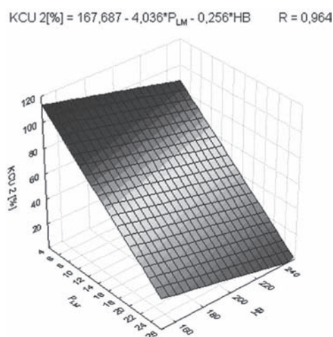
Rys. 8. Zależność uderności staliwa IN 519 od parametru Larsona-Millera i twardości Brinella rur w reformerach Z.Ch. „POLICE”
