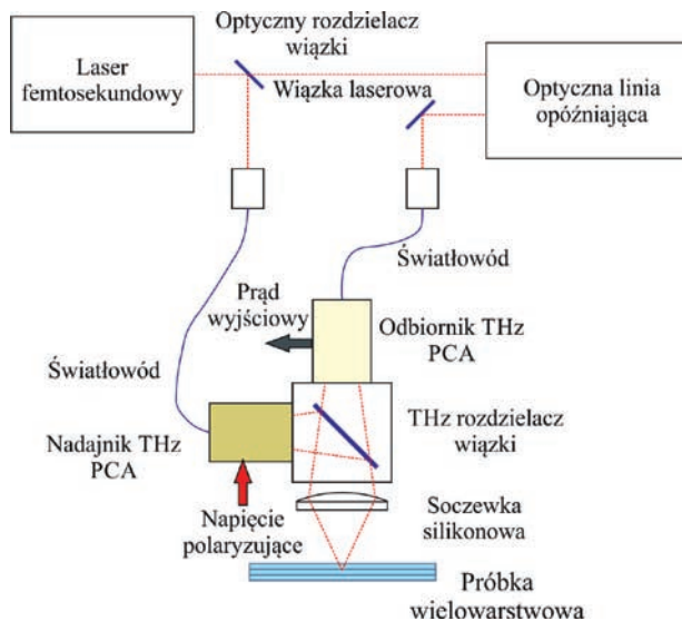
Rys. 2. Uproszczony schemat systemu teraherowego TDS pracującego w trybie odbiciowym w układzie z rozdzielaczem wiązki Fig. 2. Simplified scheme of the terahertz time domain spectroscopy working in reflection mode in configuration with beam splitter
