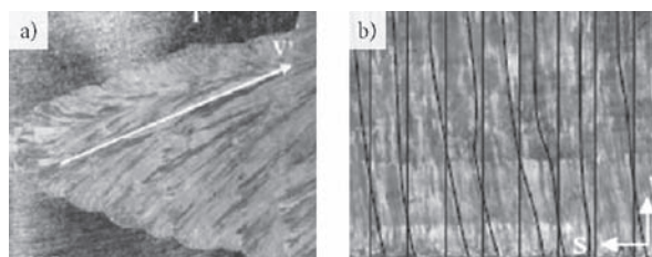
Rys. 2. Układ tekstury dendrytycznej spoiny austenitycznej w pozycji: (a) poziomej – nachylenie kryształitów około 20°; (b) pionowej – nachylenie pionowe około 90°
