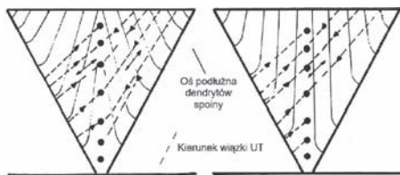
Rys. 10. Wiązka ultradźwiękowa może ulegać zniekształceniom (zagięciom) na kolumnowej niejednorodnej strukturze dendrytów, w szczególności w obszarach ich zakrzywienia (działanie podobne do fal prowadzonych – guided waves)
