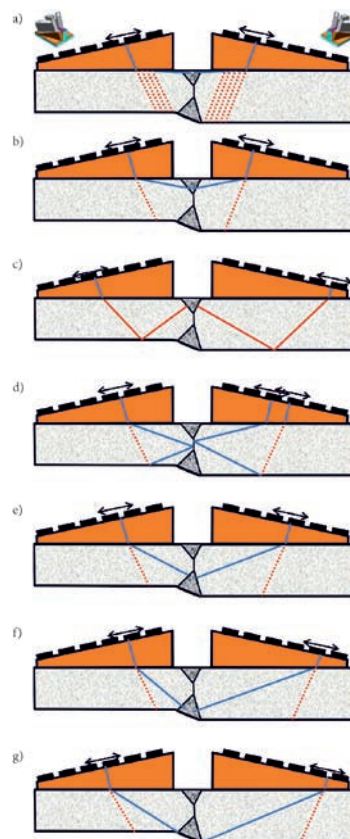
Rys. 29. Przeszukiwanie złącza głowicami PA DMA-TRL Fig. 29. Przeszukiwanie złącza głowicami PA DMA-TRL
