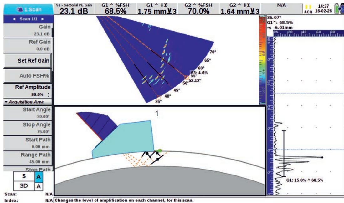
Fig. 7. Recommended Acquisition Layout; ID indication on the A-scan and Confirmed in the 3D View Rys. 7. Zalecany układ obrazowań podczas rejestracji; wskazanie na obrazie typu A i potwierdzenie w 3D
